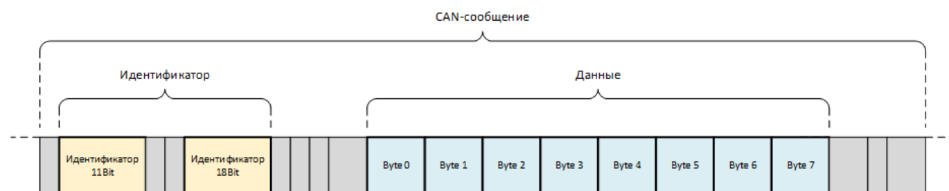
Рис. 68. Структура CAN-сообщения. Идентификатор «29 бит»
