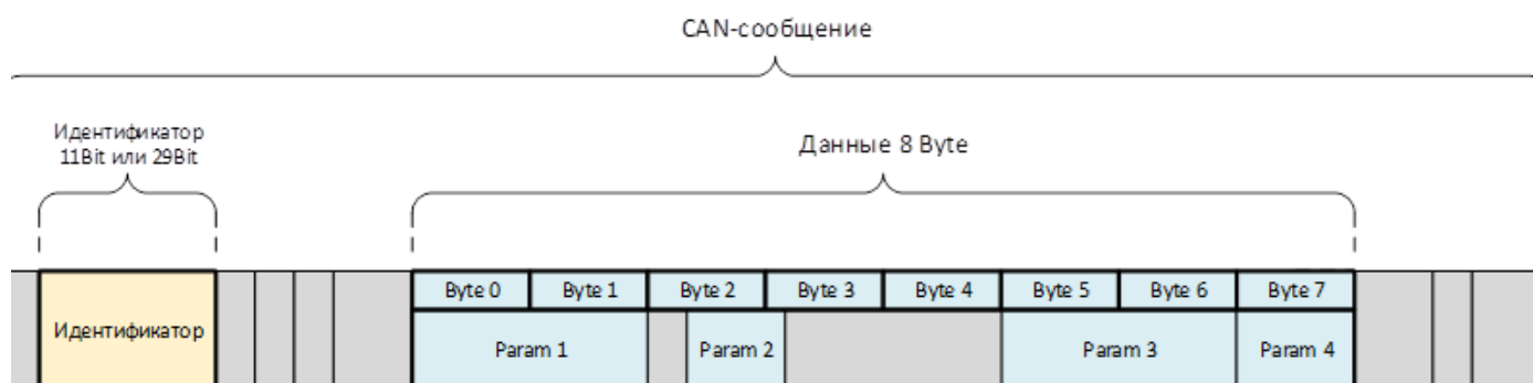
Рис. 66. Структура CAN-сообщения
