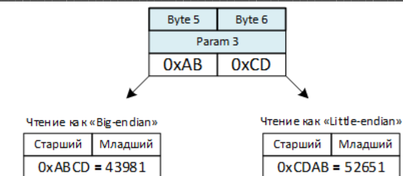
Рис. 72. Пример чтения параметра в зависимости от порядка байт
