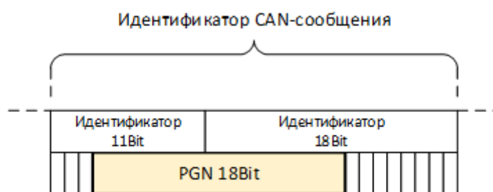
Рис. 69. Идентификатор CAN-сообщения «PGN»
